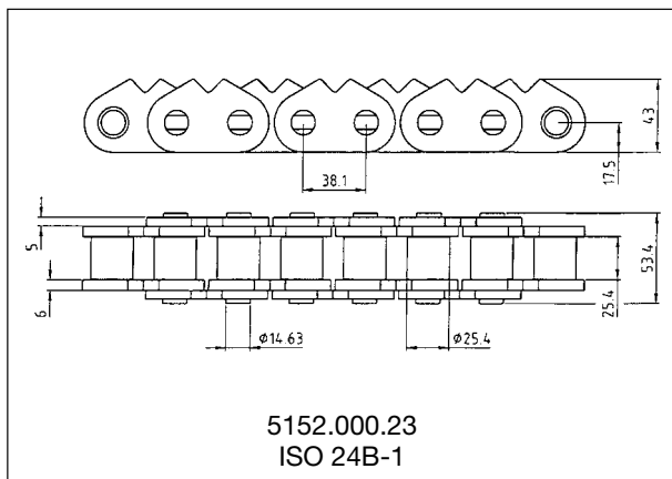
24B-1FVERZS/PLx152i
